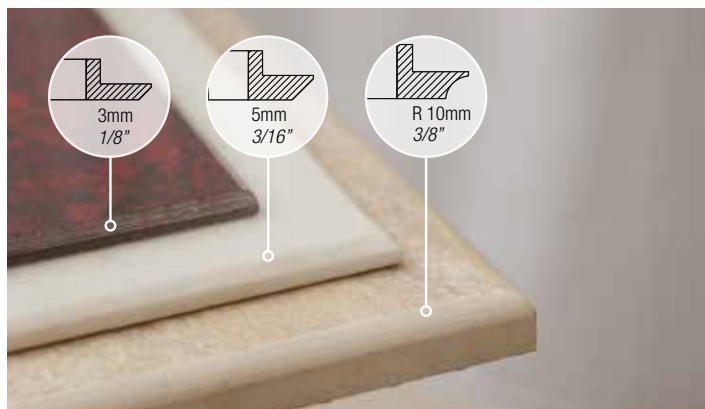
7 Protezione in policarbonato Polycarbonate protection
